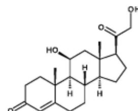
Corticosterone
