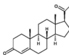
Progesterone
