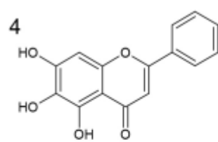
Baicalein
