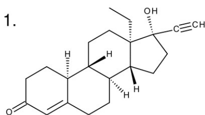
L-Norgestrel
